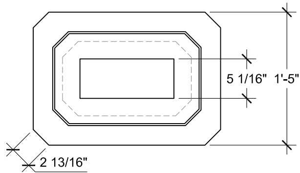
TOP VIEW SCALE: 1"= 1'-0"
